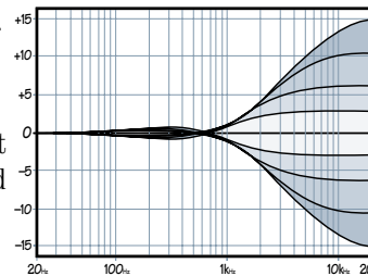
Hi EQ \pm 15\text{dB} boost/cut above 12kHz
