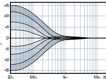
Lo EQ \pm 15\text{dB} boost/cut below 80Hz
